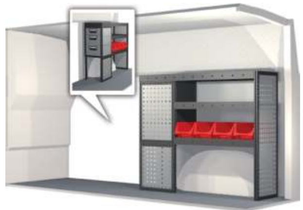
Kaluste nro: 20100130 Leveys: 999 mm Syvyys: 324 mm Korkeus: 918 mm Paino: 31.8 kg
