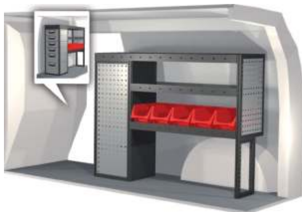
Kaluste nro: 20100162 Leveys: 1161 mm Syvyys: 324 mm Korkeus: 918 mm Paino: 42.8 kg
